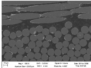
罗地亚连续纤维增强热塑性塑料扫描电子显微镜分析
